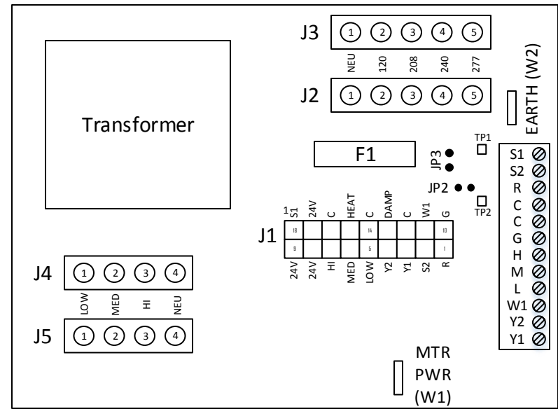
Fan Relay Board 2 - FRBii
